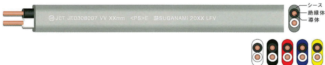
<2心ケーブル>
