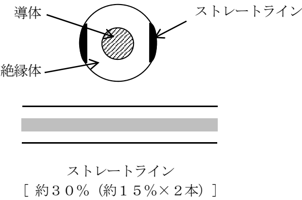
構造図
