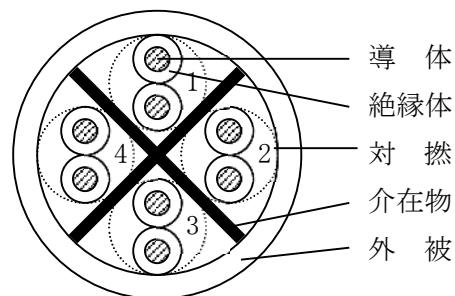
構 造 図
