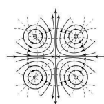
〈図1〉4心ケーブルに発生した磁界
