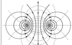
〈図2〉2心ケーブルに発生した磁界
