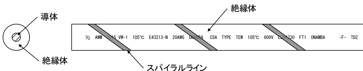
構造略図
